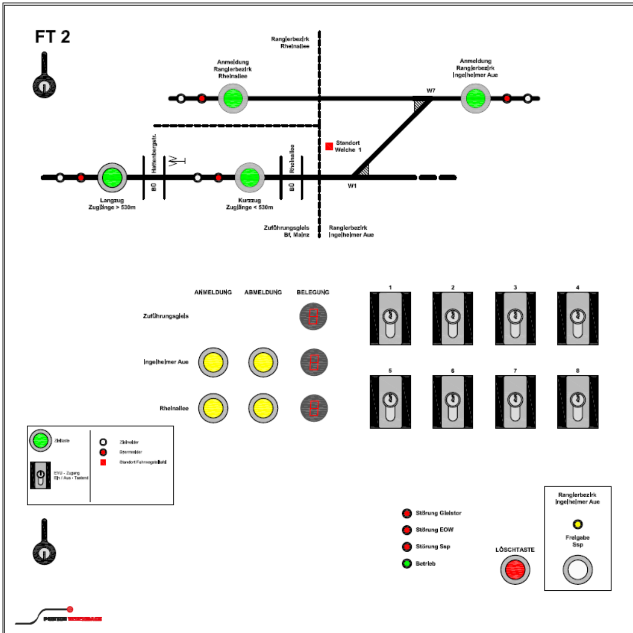
Abbildung 3 Frontansicht FT2
